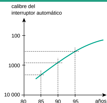
Fig. 1: Evolución de los relés electrónicos.
