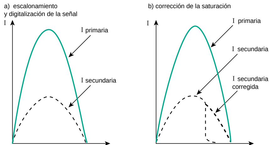
Fig. 4: Escalonamiento y corrección de la posible saturación de un TC.
