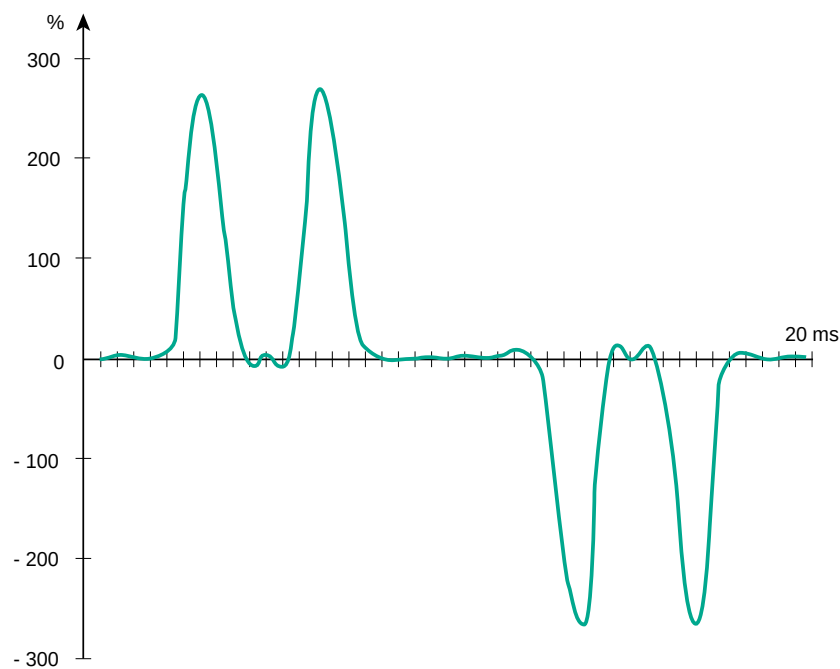
Fig. 11: Ejemplo 2: variador de velocidad de frecuencia variable.
