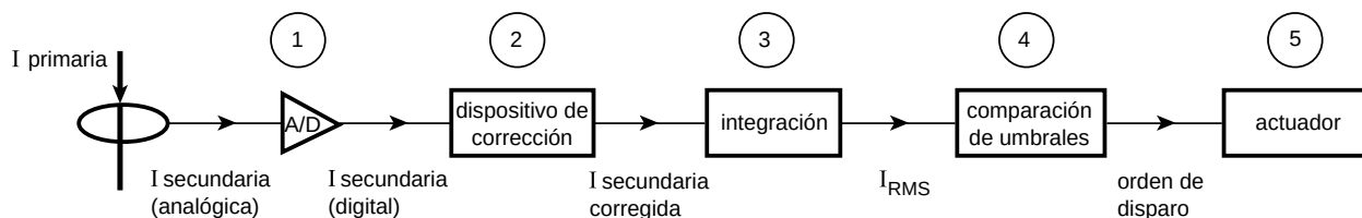
Fig. 3: Esquema funcional.
