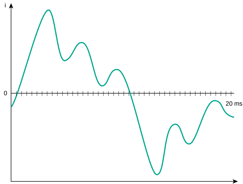
Fig. 12: Iluminación fluorescente.
