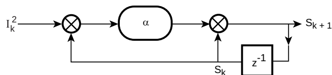
Fig. 6: Algoritmo de filtrado (R) del filtro digital de paso bajo.
