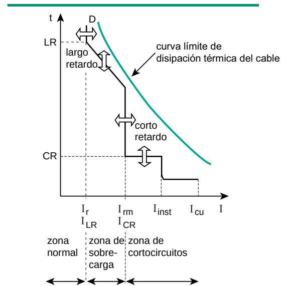
Fig. 9: Curvas de disparo de un interruptor automático electrónico.
