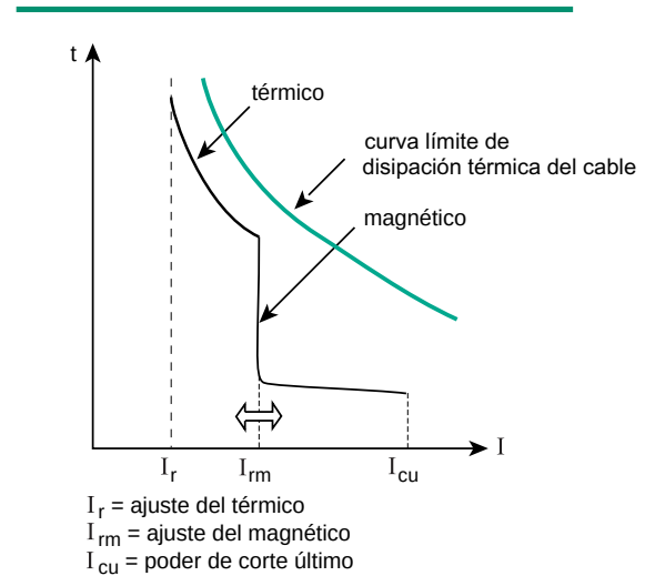
Fig. 5: Curva de disparo de un interruptor automático termomagnético.
