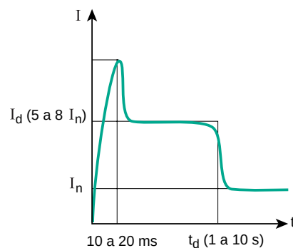
Fig. 14: Conexión de un motor.
