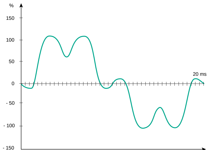
Fig. 10: Ejemplo 1: rectificador.
